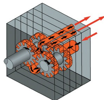
Large gamme de pompes à engrenages de précision Zenith®
